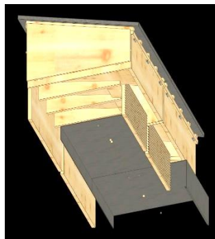
Vom CAD-Plan zur Visualisierung – Alpenglernnistkästen
